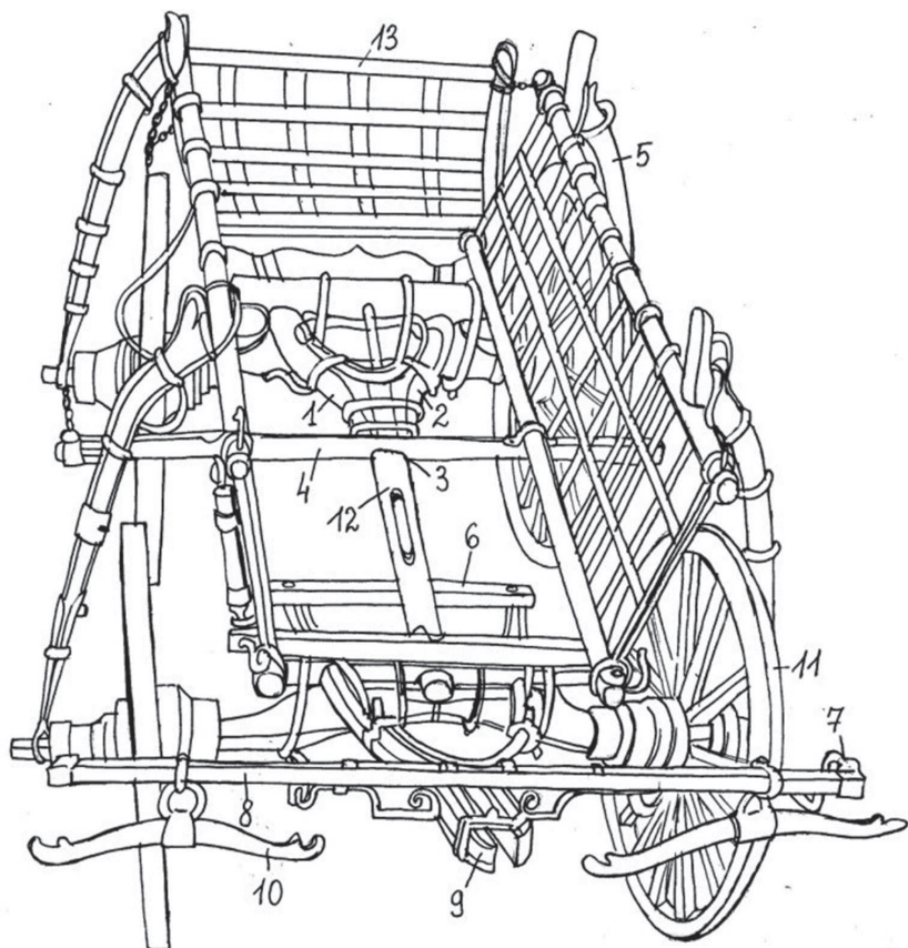
A szekér alváza: 1,2. nyújtószárny, 3. derékszög, 4. hátulsó felhérc, 5. löcs, 6. fergettyű, 7. felhércvasalás, 8. első felhérc, 9. rúdszárny, 10. hámfa, 11. szekerkerek, 12. nyújtó, 13. hátulsó saroglya. (Rajz: Kész B.)
